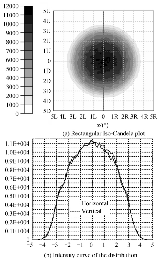
图7 面光源的发光强度分布
