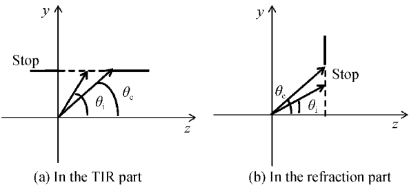
图 4 光线入射角的草图 Fig. 4 Sketch of the incident angle
