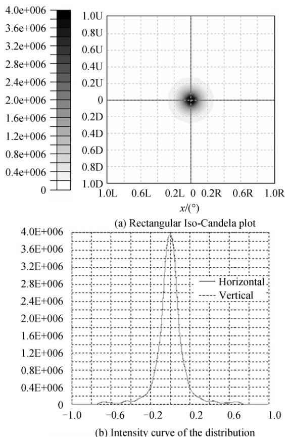
图6 点光源的发光强度分布
