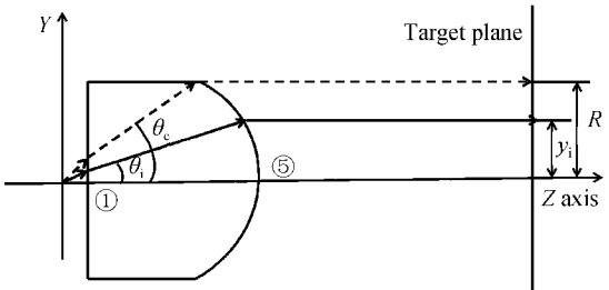
图 2 透射部分光学系统简化模型
