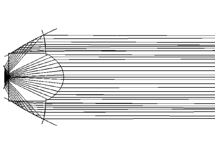
图5 ZEMAX 中模型结构图
