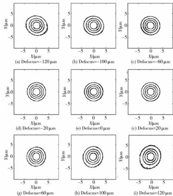
图 5 不同离焦量情况下采集的星点图像和反演得到的点扩散函数的轮廓图
