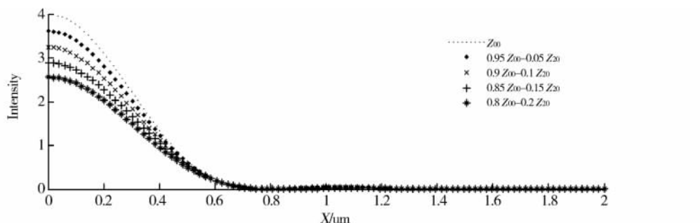
(b) 焦面处的光强分布
