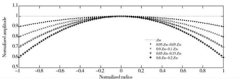
(a) 不同的出瞳振幅分布
