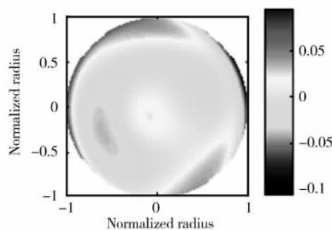
(a) 计算得到的出瞳波前拟合结果
