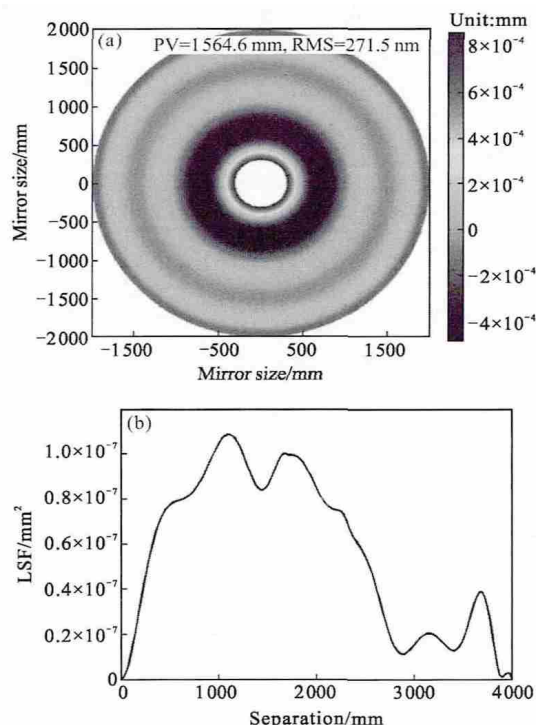
图 3 重力印透效应下反射镜面形云图和结构函数
