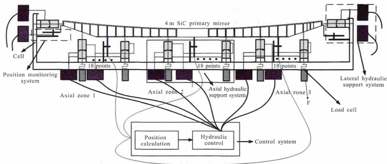
图 1 4 m 反射镜支撑系统示意图
