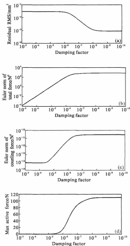
图 4 阻尼因子对主动校正力解算结果影响
