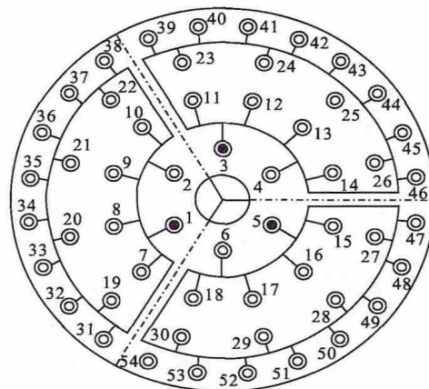
图 2 4 m 反射镜支撑点布局图
