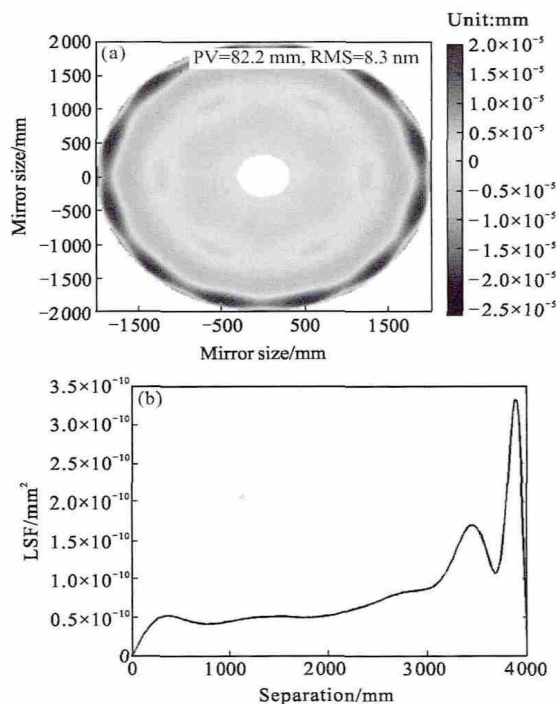
图 5 校正后的反射镜面形云图和结构函数
