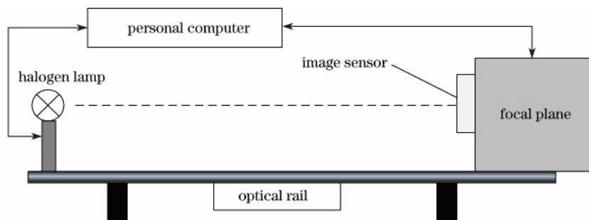
图 1 焦平面辐射定标装置示意图
