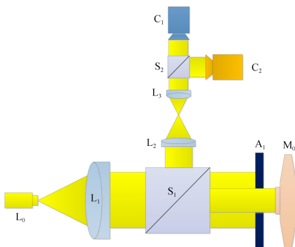
图 6 四波前剪切干涉实验光路
