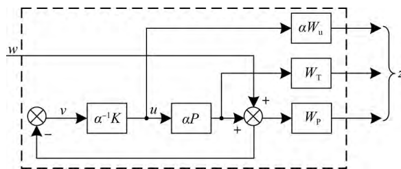
图7 扩展 H_\infty 法
