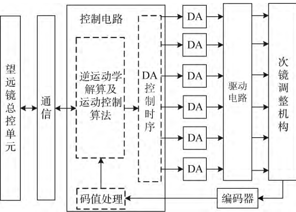
图 13 次镜六自由度调整机构控制系统图
