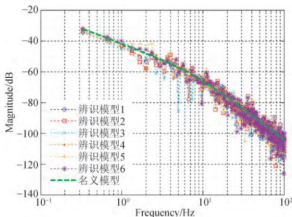
图 5 系统辨识图
