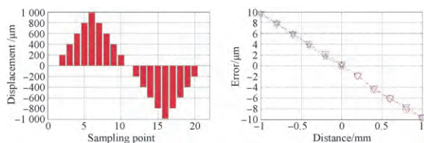
图 16 X 方向位移定位精度及误差
