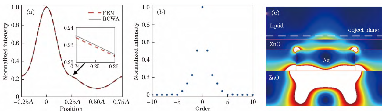
图 2 (a) k_x = |k_g| , k_y = 0 , \Delta\varphi = 0 条件下金属光栅激励起的照明条纹光强分布; (b) 照明条纹的傅里叶空间级数分布; (c) 有限元方法计算得到的金属光栅的近场光强分布
