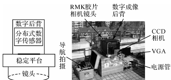
图6 基于二次成像原理的数字航摄相机系统
