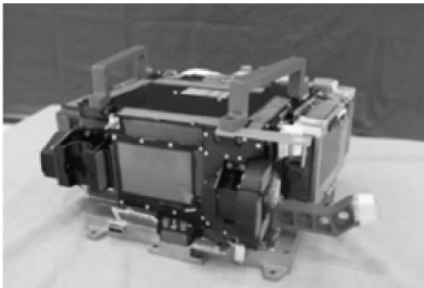
图 13 宽波段临边成像光谱仪实物照片 Fig.13 Wideband limb imaging spectrometer
