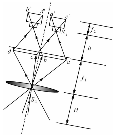
图 9 二次成像倾斜构像分析
