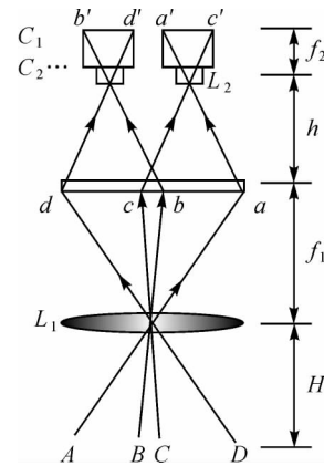
图2 数字航摄相机通用光路图
