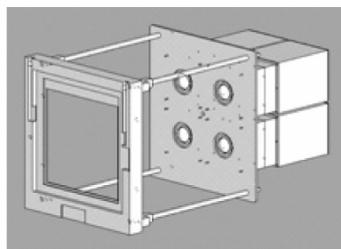
图7 数字后背结构装配体建模图
