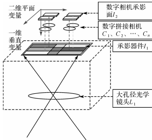
图1 通用物理模型示意
