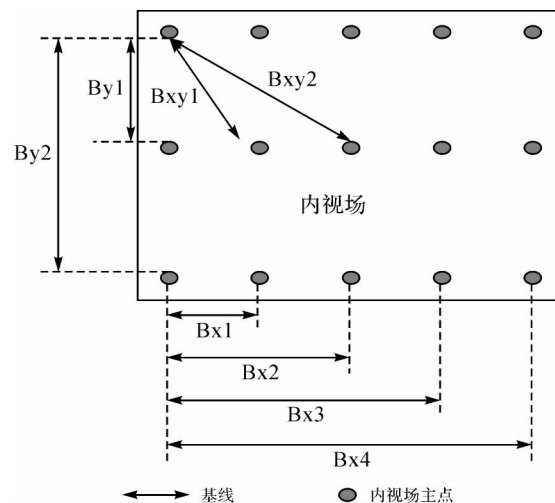
图3 内视场拼接基线形式示意图
