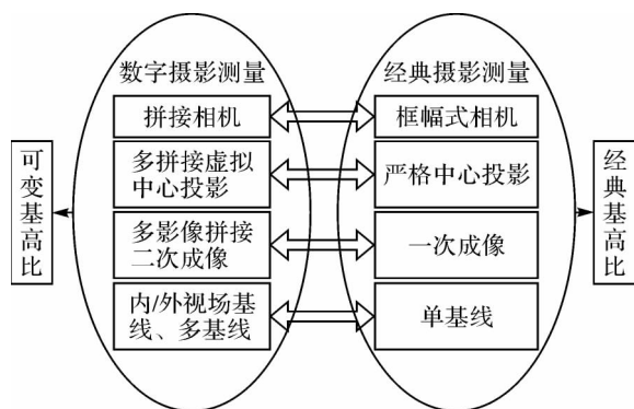
图4 数字航摄影机4大技术特征
