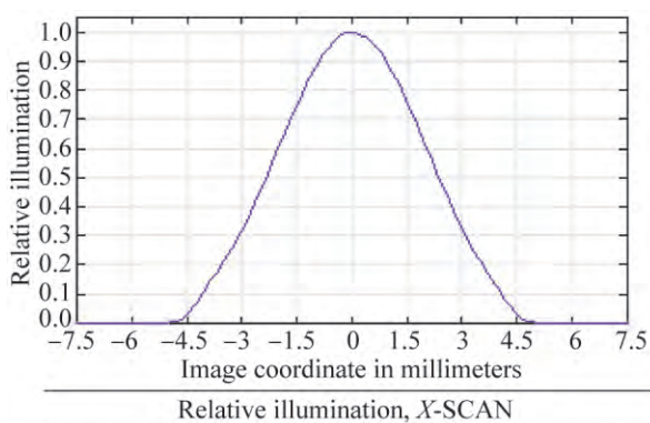
图 5 初始三反射镜系统 X, Y 方向照度图
