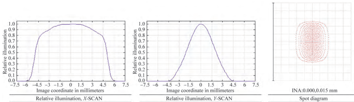
图 7 优化一圈的 X, Y 照度图及光斑图
