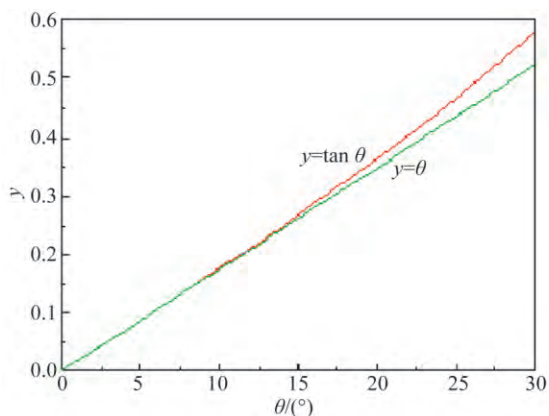
图 11 理想、实际像高与扫描角度的关系曲线
