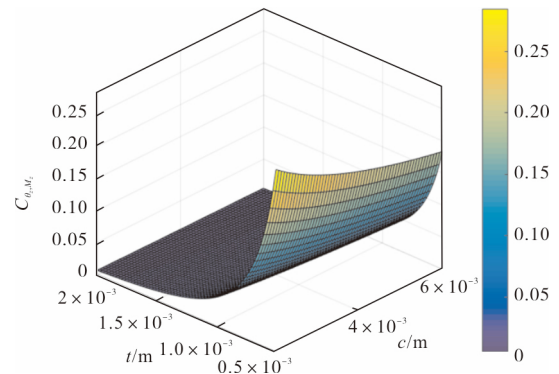
图 6 双边直圆抛物线铰链柔度 C_{\theta_z, M_z} 随设计参数 c 和 t 变化关系
