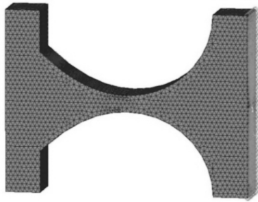
图 3 双边直圆抛物线柔性铰链的有限元模型
