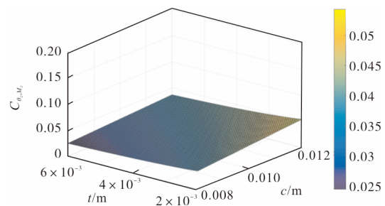
图 7 双边直圆抛物线铰链柔度 C_{\theta_z, M_z} 随设计参数 c 和 L 变化关系
