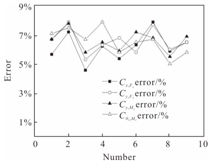
图 4 柔度理论计算结果与有限元仿真结果误差值
