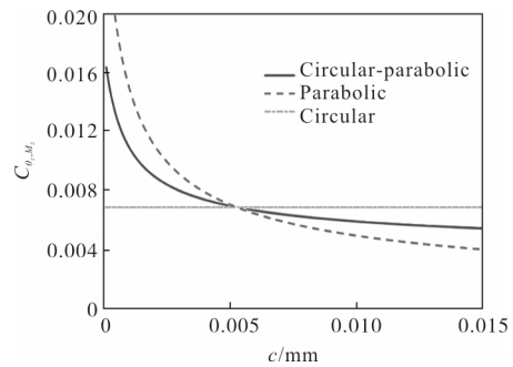
图 9 三种铰链的 C_{\theta_z, M_z} 随 c 变化关系
