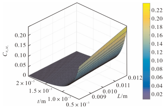
图 8 双边直圆抛物线铰链柔度 C_{\theta_z, M_z} 随设计参数 L 和 t 变化关系
