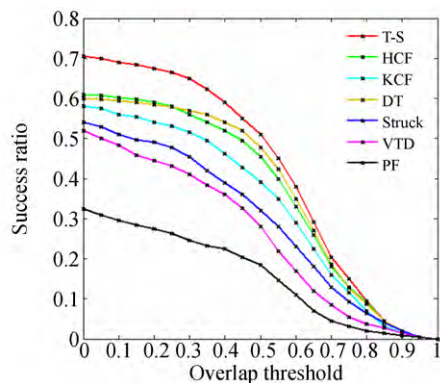
图 6 跟踪重叠率曲线
