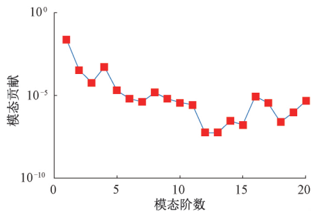
图 9 机翼模态贡献-模态阶数曲线
