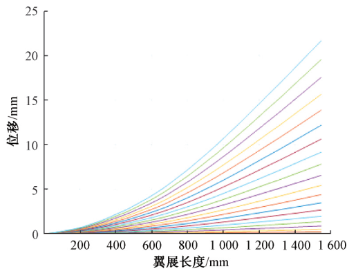
图 8 不同载荷下机翼变形曲线
