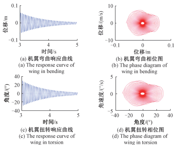
图 18 机翼的弯曲、扭转动力学响应和相位图
