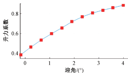
图 13 只考虑机翼刚性的气动参数
