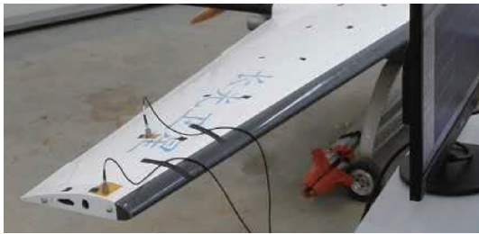
图 2 机翼模态试验
