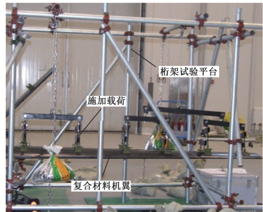
图 10 机翼静载试验
