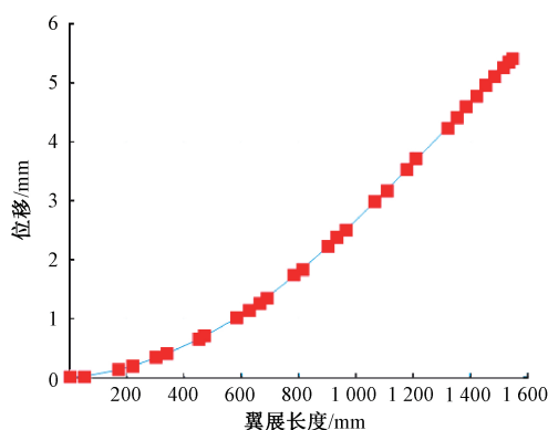
图 7 机翼变形曲线
