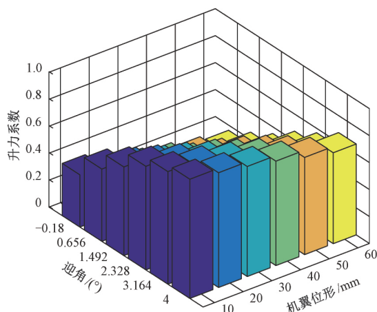
图 14 考虑机翼柔性的气动参数
