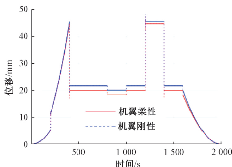
图 17 翼尖位移结果对比
