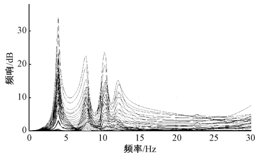
图 4 第 4 点的 FRF 计算结果
