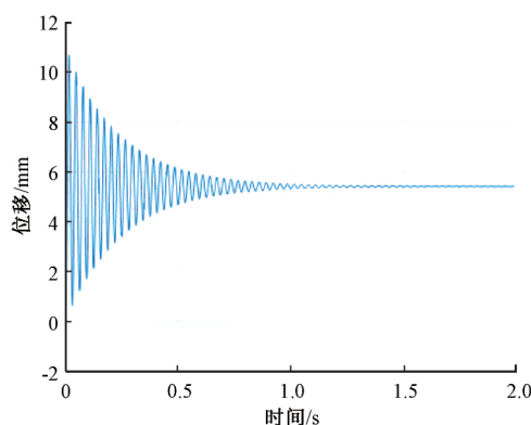
图 6 翼尖位移曲线
