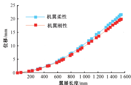
图 15 机翼变形结果对比
