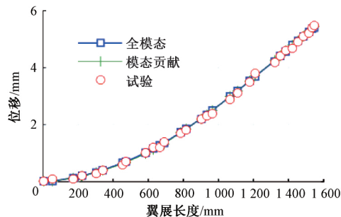
图 12 机翼变形结果对比
