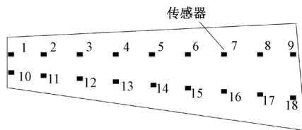
图 3 模态试验传感器布局
