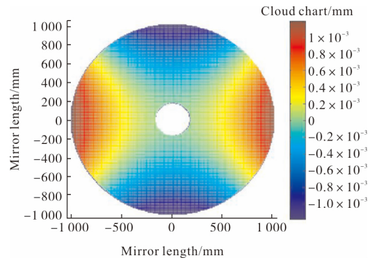
图 5 像散面形云图
