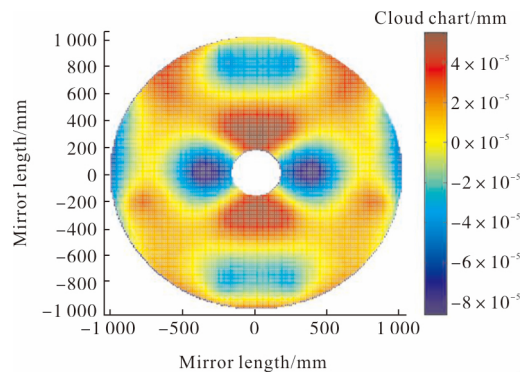
图 6 校正后的主镜面形云图
