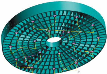
图 3 有限元分析模型 Fig.3 Finite element analysis model
