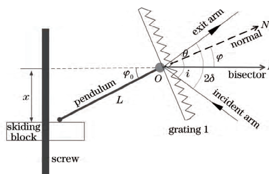
图1 波长线性扫描机构示意图
