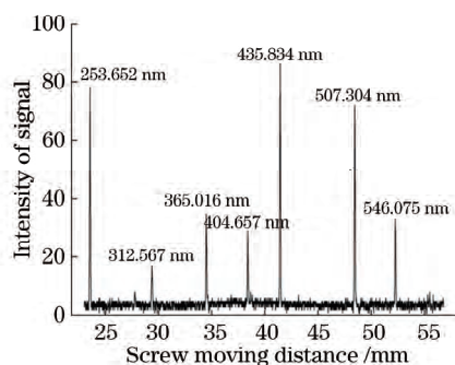
图 5 汞灯光源照明可见光通道的输出信号曲线
