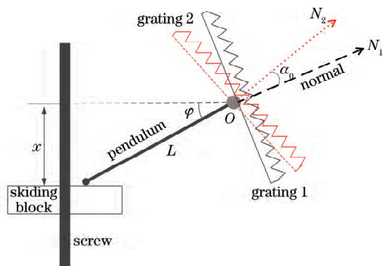
图2 双通道光栅光谱仪波长扫描机构示意图
