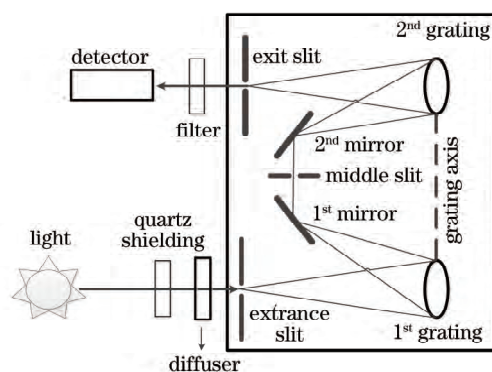
图4 每个通道的工作原理图
