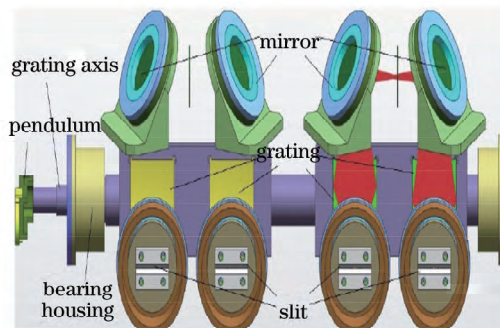
图3 太阳辐射度光谱仪结构图
