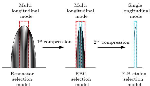
图1 选模原理图
