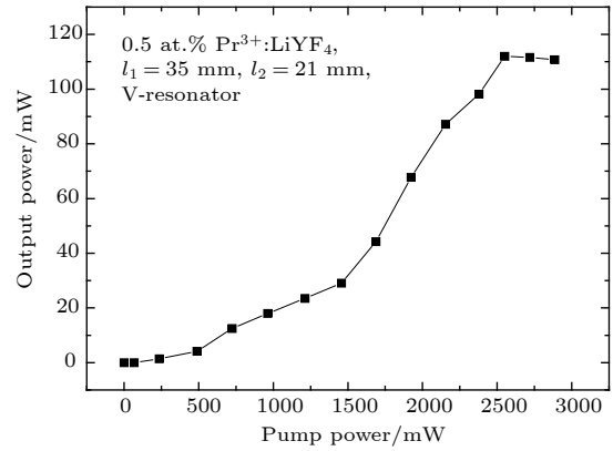
图8 360 nm 单纵模激光输出功率相对于入射抽运功率 (444 nm 与 469 nm 合束) 的变化
