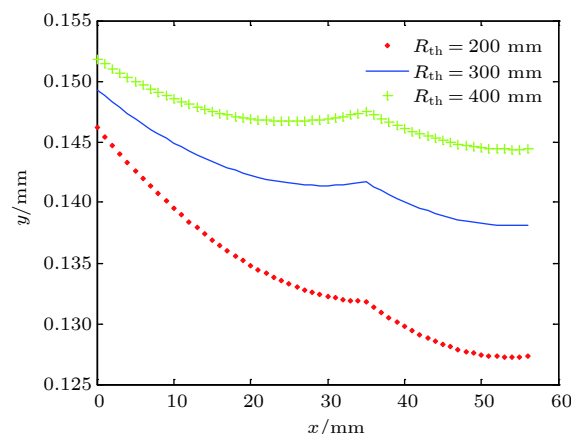
图 6 晶体热焦距 R_{\text{th}} 分别为 200, 300, 400 mm 时, \text{Pr}^{3+}:\text{LiYF}_4 和 LBO 晶体内束腰半径随着 LBO 晶体与 M1 之间距离的变化情况
