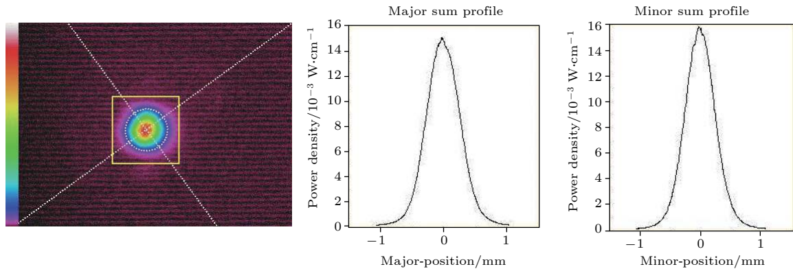
图9 远场光斑
