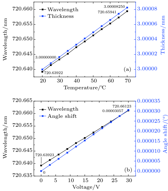
图7 720 nm 激光中心波长调谐 (a) 中心波长随 F-P 标准具温度及厚度的变化; (b) 中心波长随 PZT 电压及 F-P 标准具角度的变化
