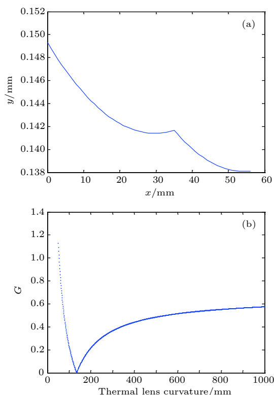
图 5 谐振腔稳定性分析 (a) 晶体热焦距 R_{\text{th}} 取 300 mm 时, 腔内两个束腰半径模拟图; (b) 谐振腔稳定参数 G 随热焦距 R_{\text{th}} 的变化
