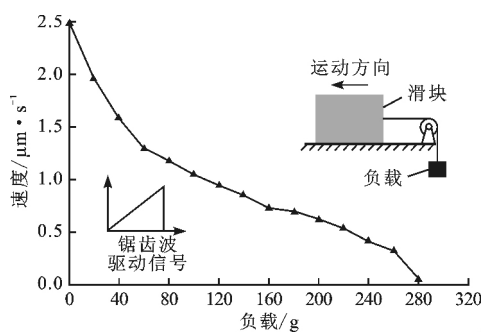
图11 100 V、10 Hz条件下驱动器输出速度与负载的关系
