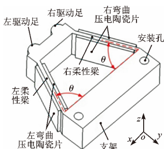
(b) 定子三维模型
