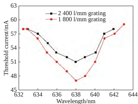
图5 两种不同刻线密度下光栅外腔半导体激光器阈值电流随激射波长的变化
