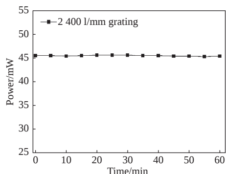
图 7 光栅外腔半导体激光器的输出功率稳定性测试结果
