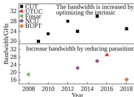
图 6 VCSEL 带宽进展
