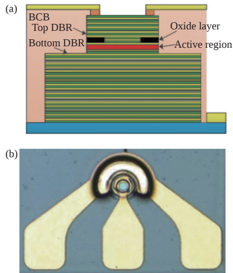
图 5 (a) 高速 VCSEL 的横截面示意图, (b) 已制备完成的 VCSEL 显微镜图像 [24]
