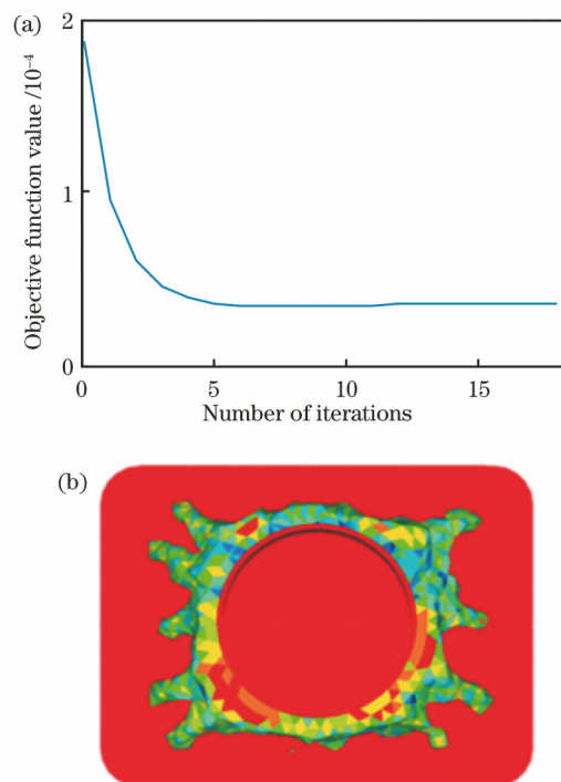
图 4 迭代收敛曲线及优化结果。(a) 迭代收敛曲线; (b) SIMP 拓扑优化结果
