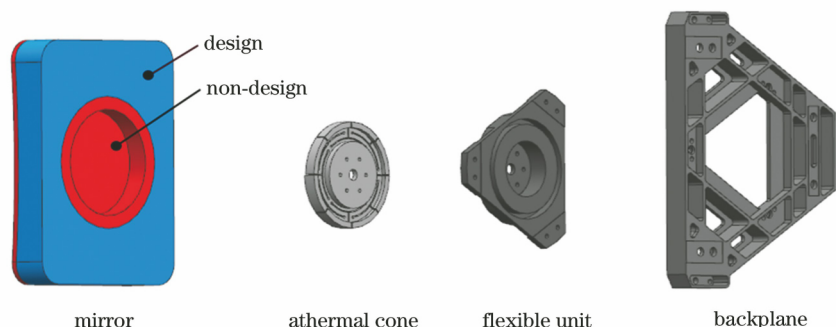
图 2 原始反射镜的组件结构
