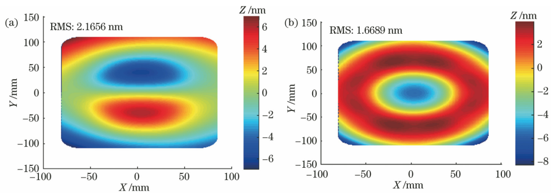
图 8 不同情况下的面形分析结果。(a) x 方向重力; (b) 4\text{ }^{\circ}\text{C} 温升
