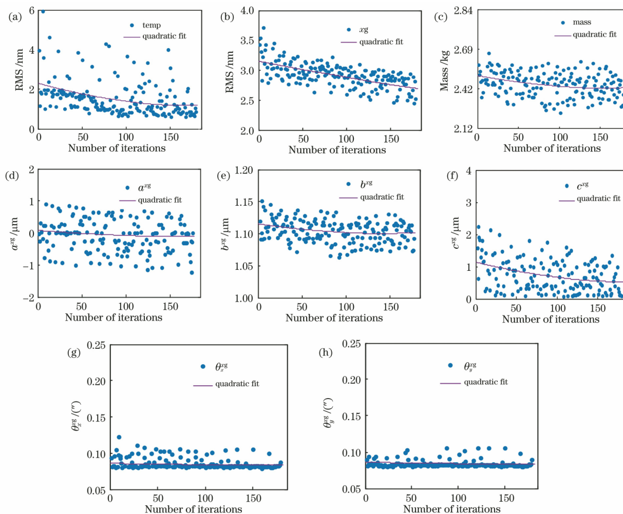
图 7 不同情况下优化后的迭代曲线。(a) +4\text{ }^{\circ}\text{C} 温度面形 RMS 值;(b) x 方向重力面形 RMS 值;(c)反射镜组件质量;(d)重力工况 x 方向偏心;(e)重力工况 y 方向偏心;(f)重力工况 z 方向偏心;(g)重力工况 x 方向倾斜;(h)重力工况 y 方向倾斜
