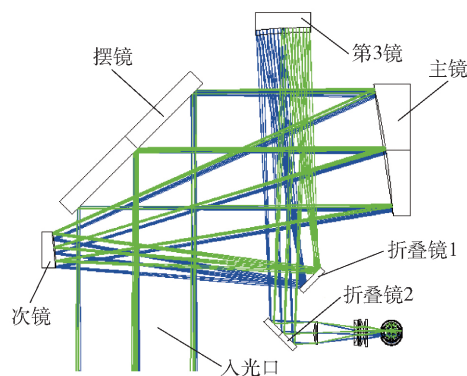
图 1 某相机光学设计图
