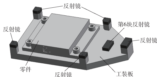
图 3 加工检测工装与调整垫图
