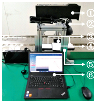
图 6 高光谱图像采集系统 Fig 6 The acquisition system of hyperspectral image
