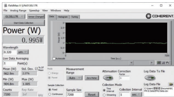
图 6 320 nm 紫外激光功率稳定性
