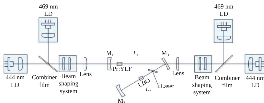
图 3 腔型结构图
