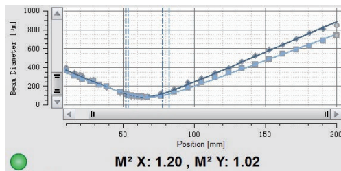
图 8 光束质量因子 ( M^2 )
