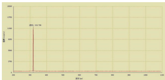
图 5 320 nm 紫外光光谱测试
