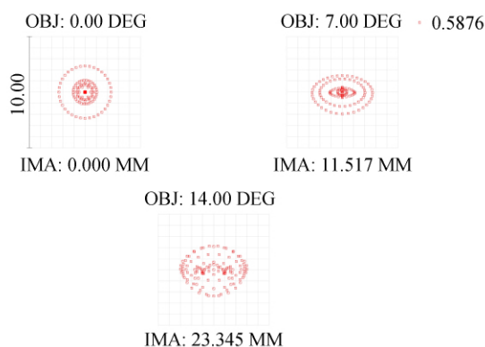
图8 光学系统点列图设计值
