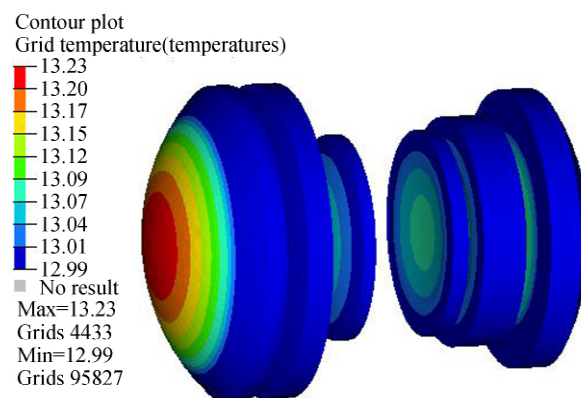
图4 工作10 min时透镜温度分布
