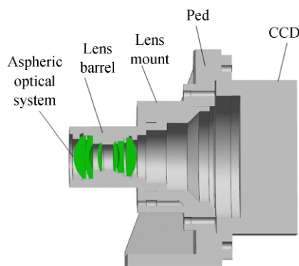
图1 机载相机三维结构
