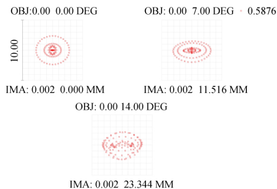
图9 开始工作时点列图拟合值
