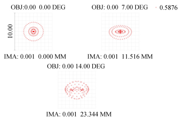
图 13 工作 40 min 点列图拟合值
