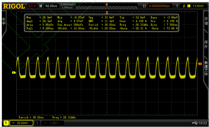
图5 室温下，泵浦功率为4.5W时， \text{Cr}^{4+} :YAG被动调Q的VECSEL输出的脉冲波形
