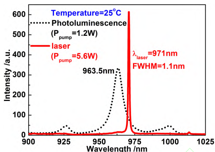
图2 室温下，1.2W泵浦时增益芯片的荧光谱，以及5.6W泵浦时VECSEL的激光光谱
