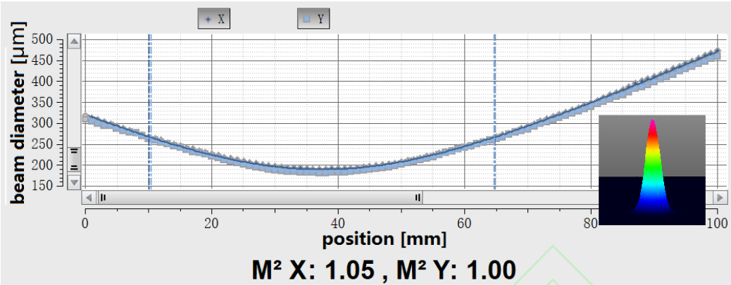
图4 924mW输出功率时，激光束的 M^2 因子。右下插图为光强分布的三维图
