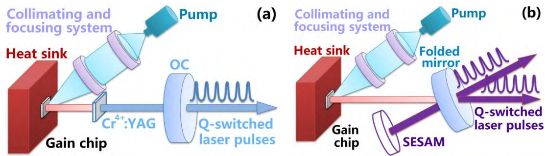
图1 被动调Q的VECSELs实验示意图。(a) Cr 4+ :YAG晶体被动调Q的VECSEL; (b) SESAM被动调Q的VECSEL
