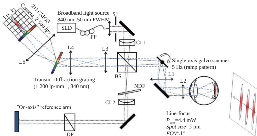
图 3 线场谱域 OCT 的原理图 [39]
