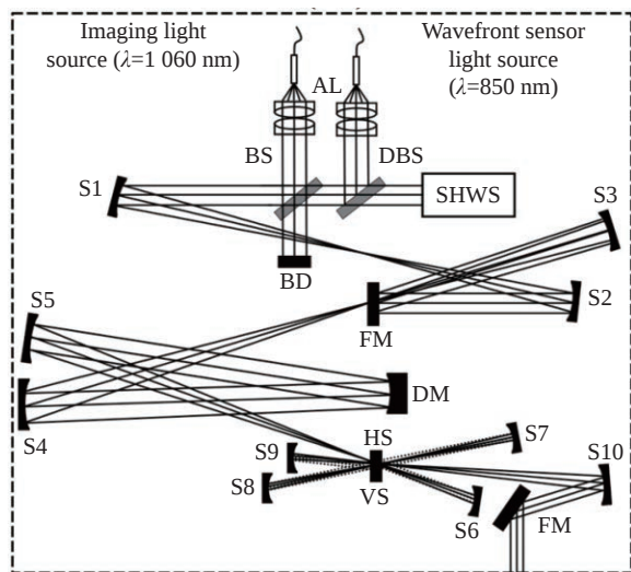
图 4 AO 扫描系统光学原理图 [54]
