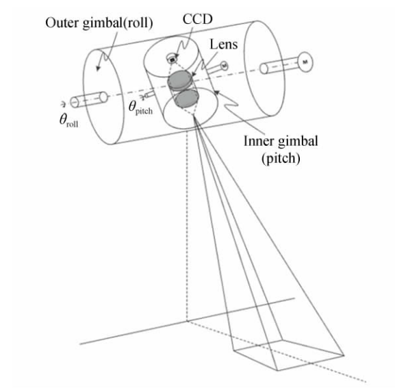
图1 航空相机结构示意图
