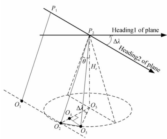
图 4 航向角变化对重叠率影响
