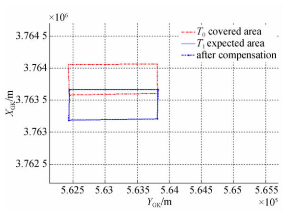
图8 飞机姿态角影响补偿结果
