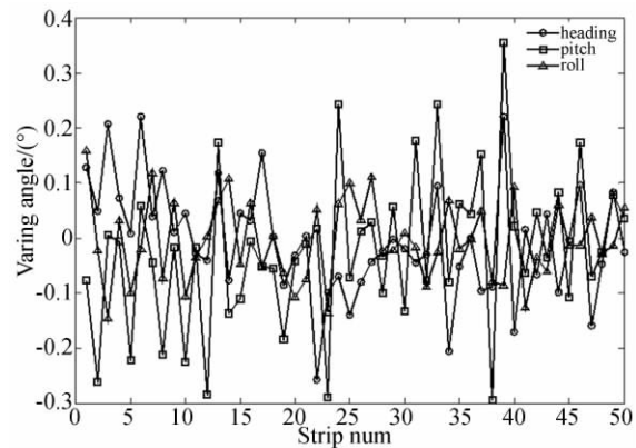
图 10 飞机姿态角波动
