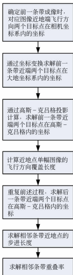
图 3 重叠率计算流程
