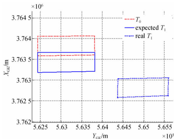
图 7 载机姿态角综合影响
