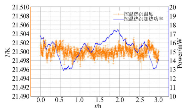
(a) 控温热沉温度及加热功率
