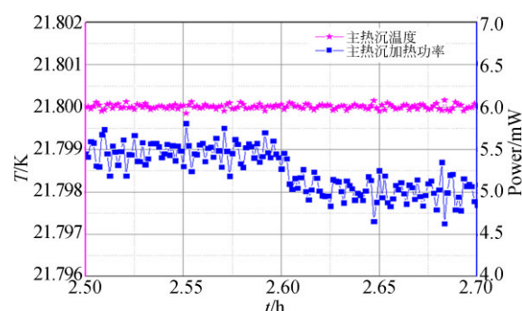
(b) 主热沉温度及加热功率
