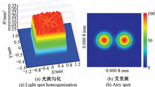
图4 匀化系统及光学分辨率仿真结果
