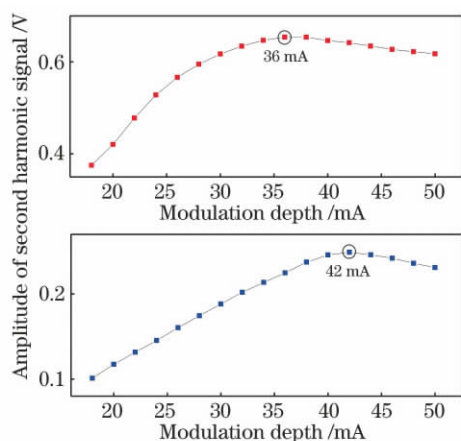
图 7 不同调制电流幅值下解调的 \text{CH}_4 和 \text{CO}_2
