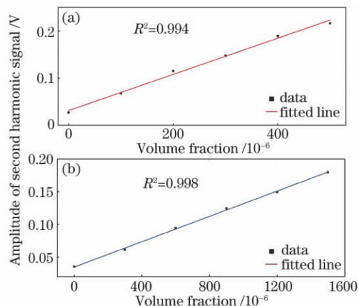
图 9 \text{CH}_4 和 \text{CO}_2 二次谐波信号幅值与对应浓度的关系。
