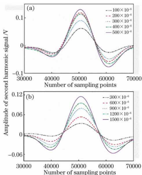
图 8 不同浓度 \text{CH}_4 和 \text{CO}_2 的二次谐波
