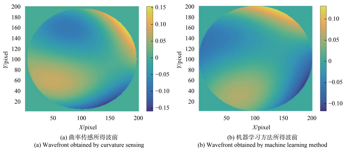
图 12 重建低阶波前对比
