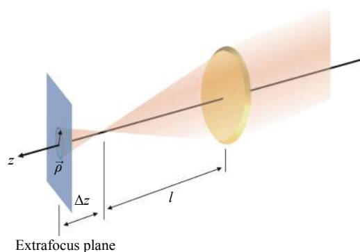
图 1 曲率传感原理图
