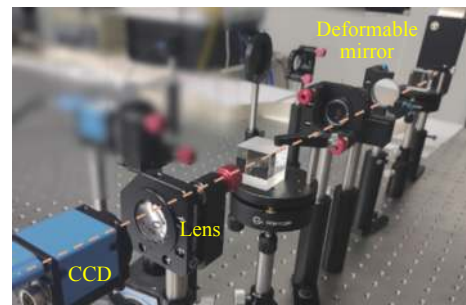
图 9 大范围曲率传感实验装置图
