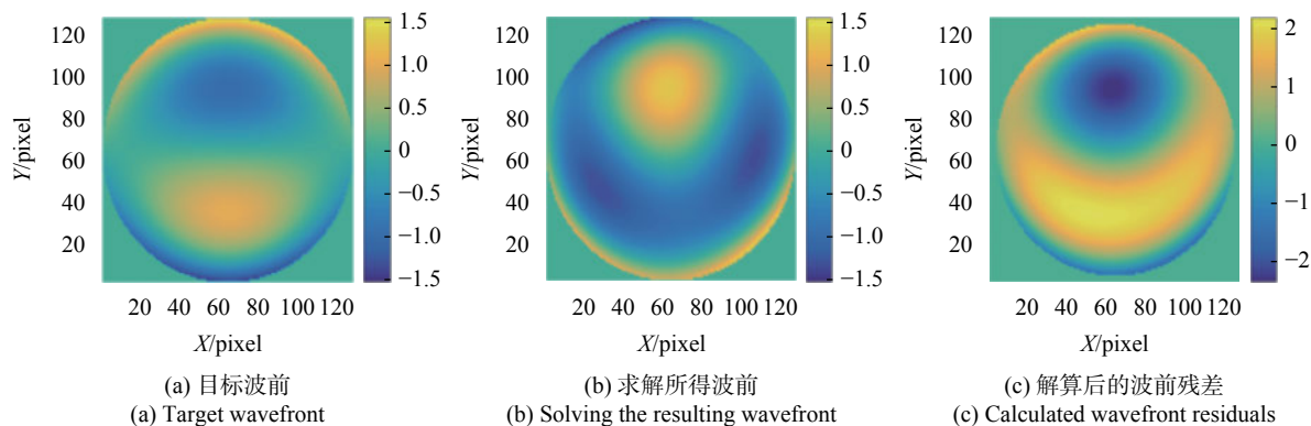
图 6 多重离焦主导波前重建精度图 (以波前 RMS 变化为准)
