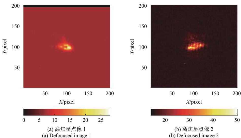
图 11 离焦主导波前焦前焦后光强分布
