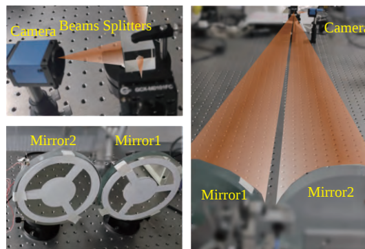
图 4 曲率传感实验现场图
