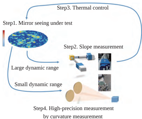
图 1 镜面视宁度测量过程图
