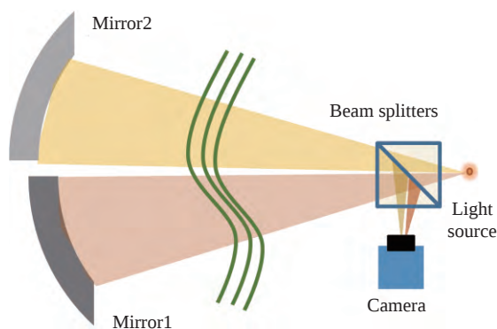
图 3 曲率传感实验示意图
