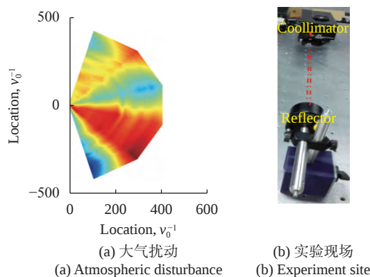
图 2 基于斜率的波前检测
