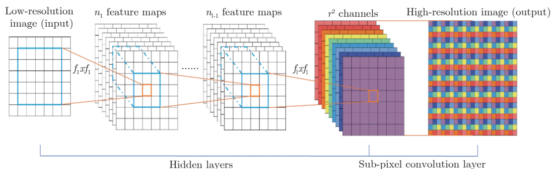
图 6 ESPCN 网络结构 [33]
