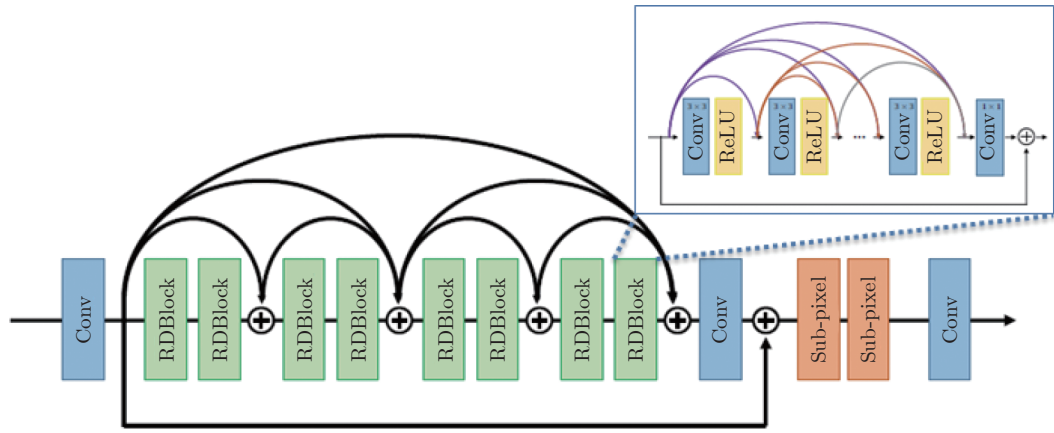
图 13 NatSR 网络结构 [45] Fig.13 The NatSR network structure [45]
