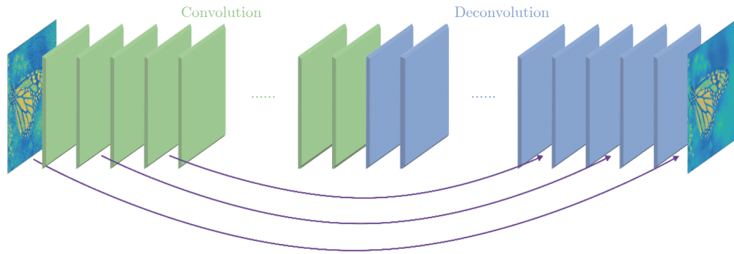
图 7 RED-Net 结构 [34]
