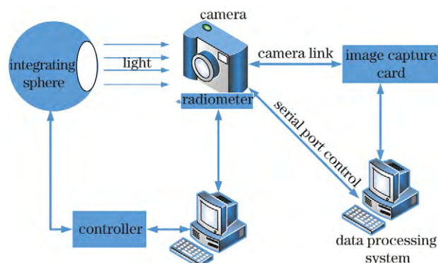
图 6 图像采集系统的原理
