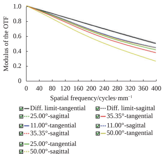
图 4 MTF 曲线图
