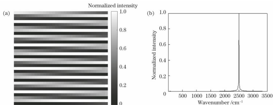
图7 当 h_1 = 1.06 \mu\text{m} , M = 6 时,仿真得到的基于微反射镜的马赫-曾德尔干涉系统的干涉图和频域光谱图。
