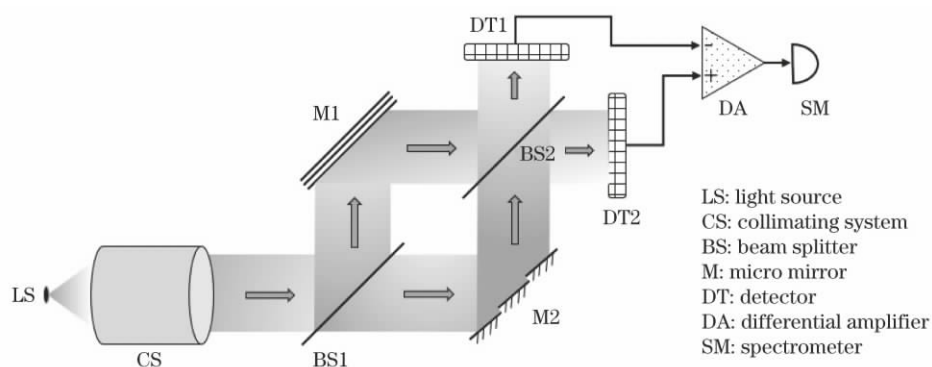
图 1 新型静态 FTS 示意图
