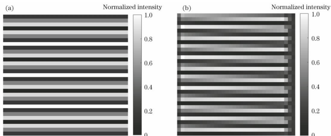
图 3 当 h_1 = 1.06\text{ }\mu\text{m} 时, 基于微反射镜的马赫-曾德尔干涉系统的干涉图。
