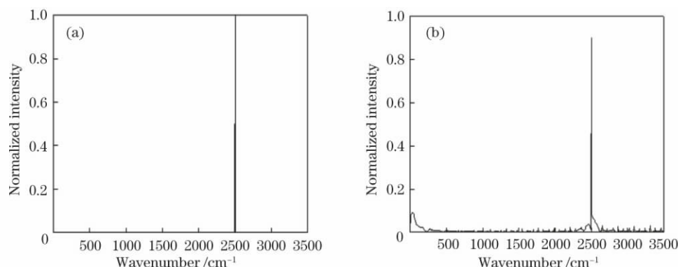
图 4 当 h_1 = 1.06 \mu\text{m} 时,基于微反射镜的马赫-曾德尔干涉系统的频域光谱图。
