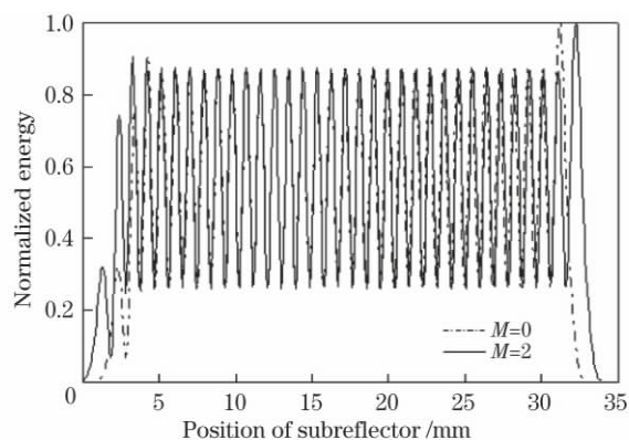
图6 第二个微反射镜 M_2 上各子反射面反射的能量分布
