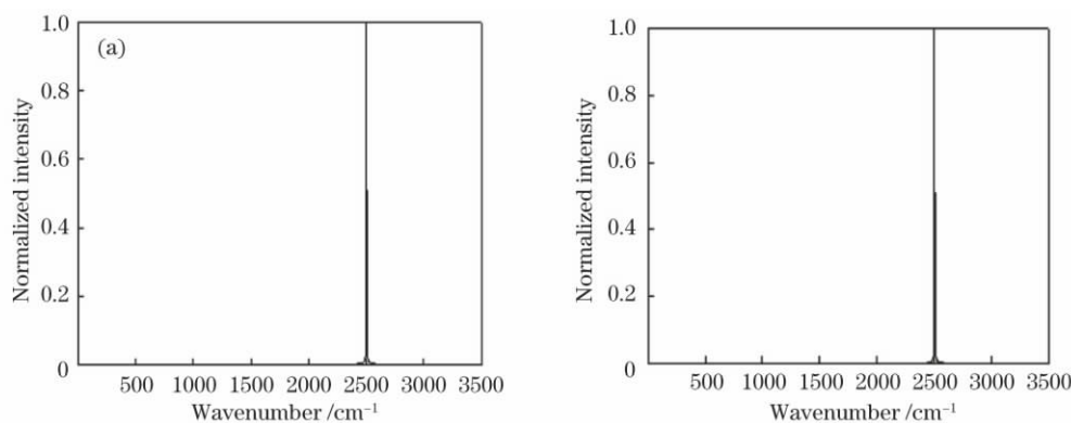
图8 当 h_1 = 0.5 \mu\text{m} , M = 6 时,基于微反射镜的马赫-曾德尔干涉系统的频域光谱图。(a)理想频域光谱图;
