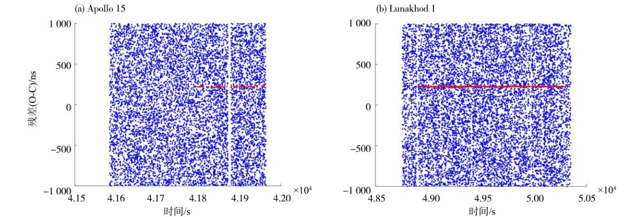
图 3 Apollo 15 和 Lunakhod 1 角反射器回波信号残差 Fig. 3 Apollo 15 and Lunakhod 1 corner reflector echo signal
