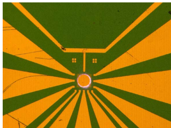
图 2 2×2 超导阵列探测器
