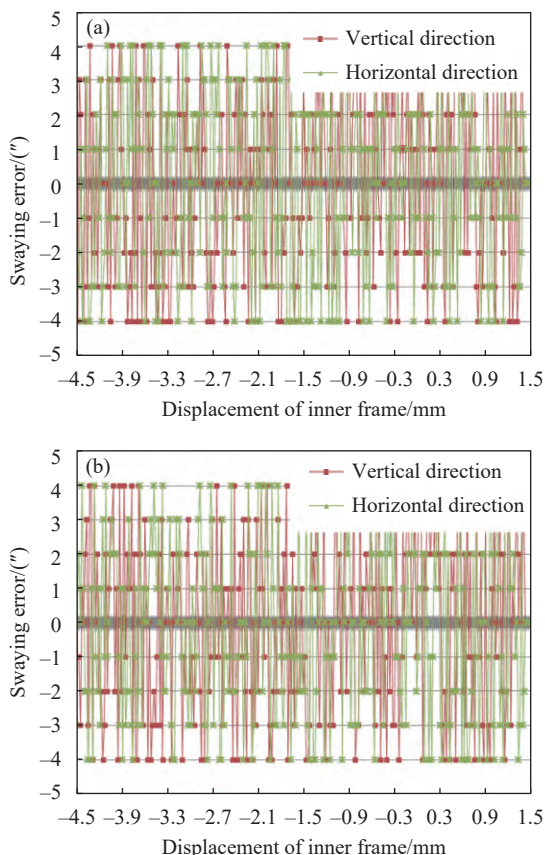
图 7 步进电机 (a) 正转和 (b) 反转时调焦机构晃动精度曲线图
