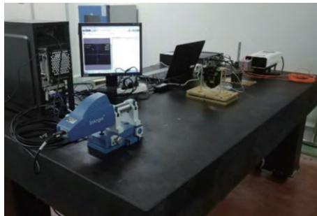
图 5 实验场景图
