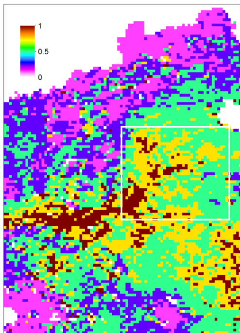
(g)201909 AOD_f\_aver
