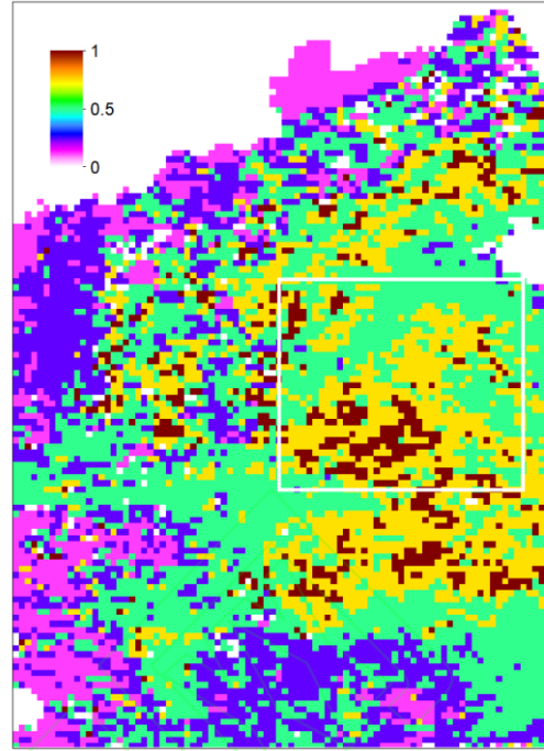
(d)201906 AOD_f\_aver
