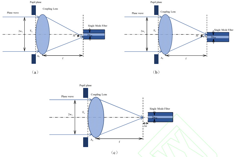
图2 对准误差示意图
