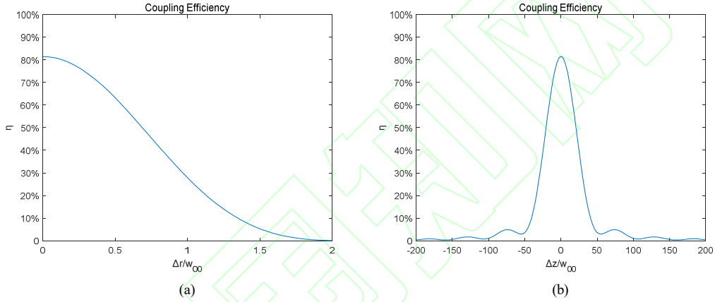
图 3 耦合效率随对准误差变化曲线
