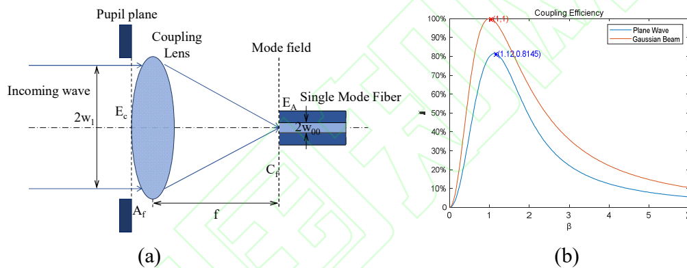
图1 理想条件下单模光纤耦合
