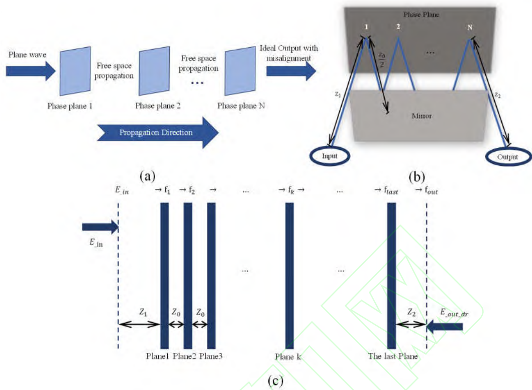
图 4 MPLC 示意图
