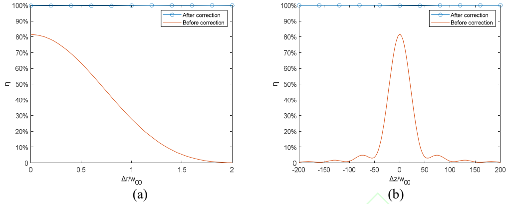
图 10 MPLC 校正前后耦合效率曲线
