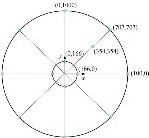
图 5 主镜采样位置
