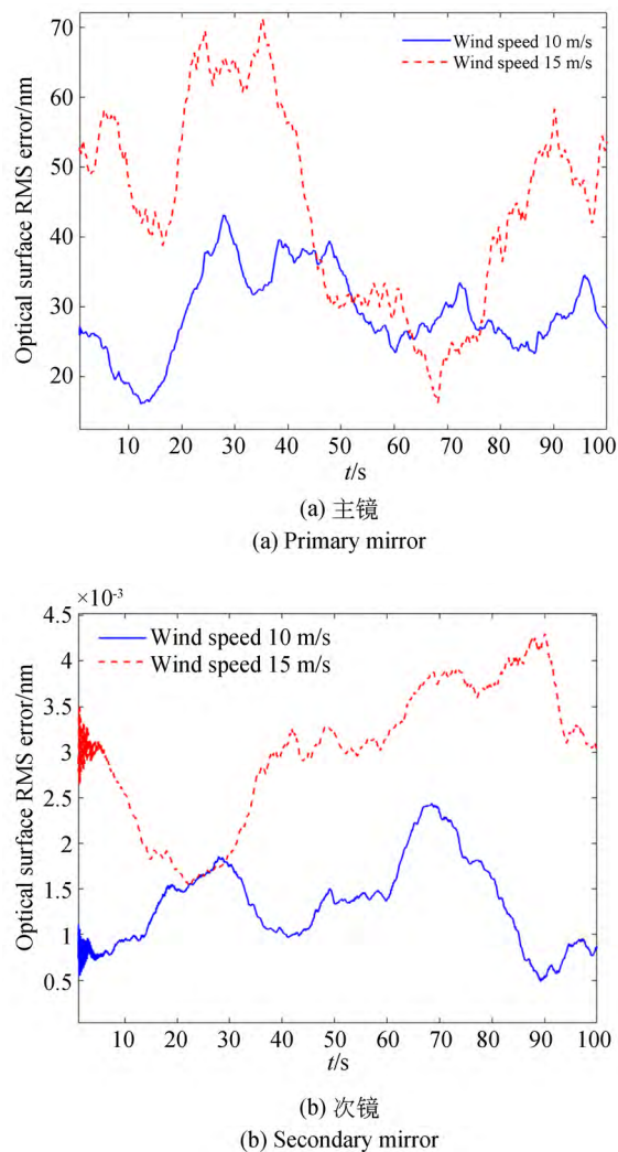
图 7 主镜和次镜镜面面形精度-主镜单独加载
