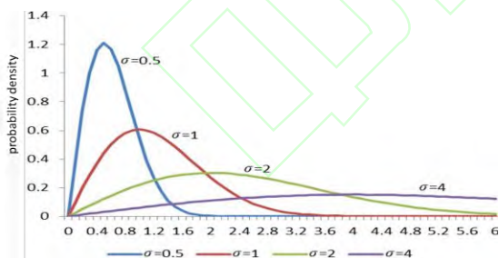
图 3 典型瑞利分布概率密度曲线图
