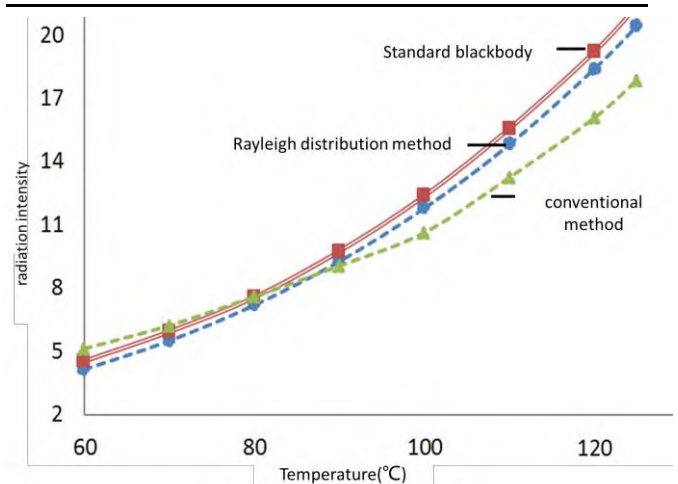
图7 不同方法反演精度比对
