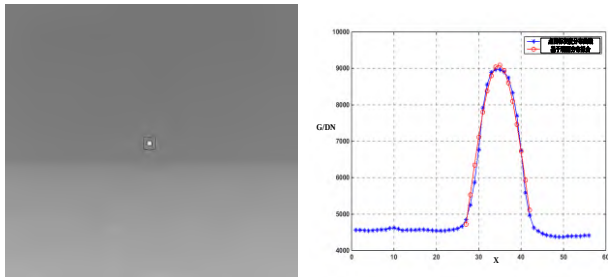
图5 实验中红外目标图像及瑞利分布拟合情况
