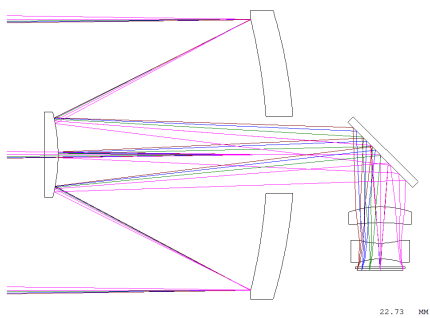
图 3 光学设计方案
