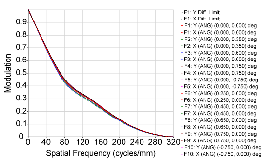
图 4 MTF 曲线
