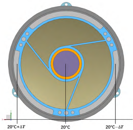
图 7 梯度温度分布
