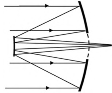
图1 同轴双反光学系统
