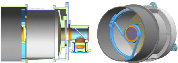
图 6 整体光机结构图
