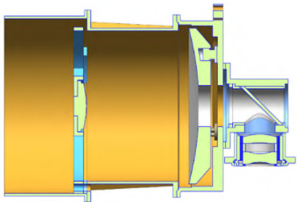
图 8 对比方案的结构形式
