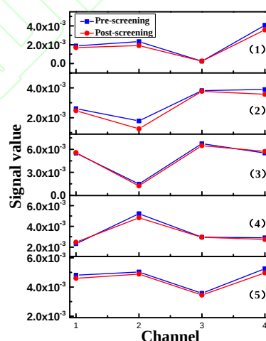
图4 筛选试验前后暗电流对比
