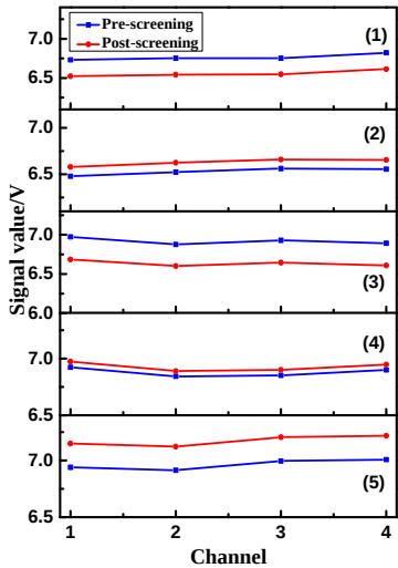
图 5 筛选试验前后信号响应度对比
