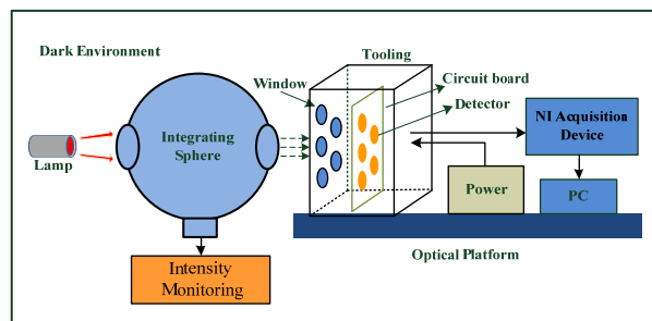
图 1 筛选系统的结构框图
