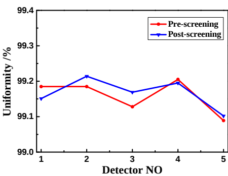
图 6 筛选试验前后响应度均匀性对比
