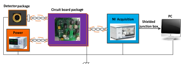
图3 抗干扰设计框图
