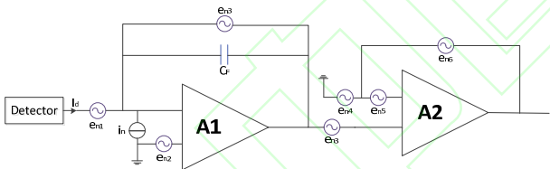
图 2 电路噪声分析模型
