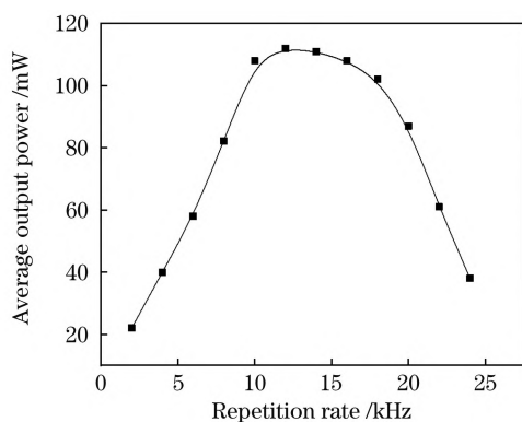
图 7 不同频率下的输出功率
