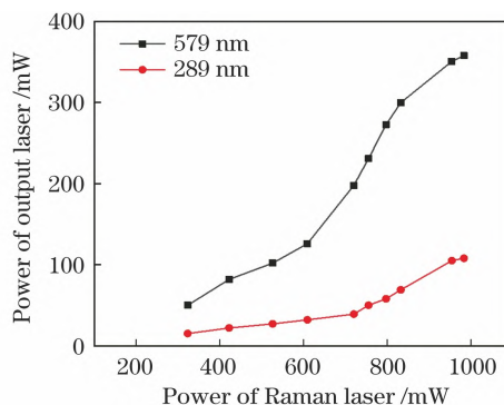
图6 二倍频光及紫外光输出功率曲线
