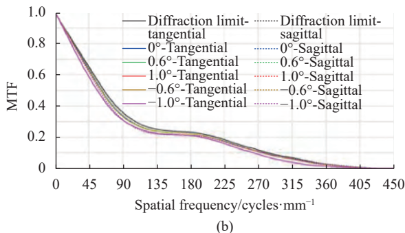
图 5 2° 视场包含两片校正镜的折反射光学系统。(a) 布局图; (b) MTF 图
