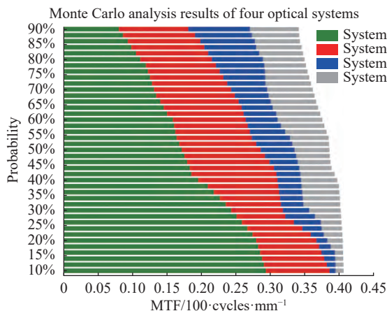
图 10 “系统 1”至“系统 4”的 MTF 蒙特卡洛分析结果图
