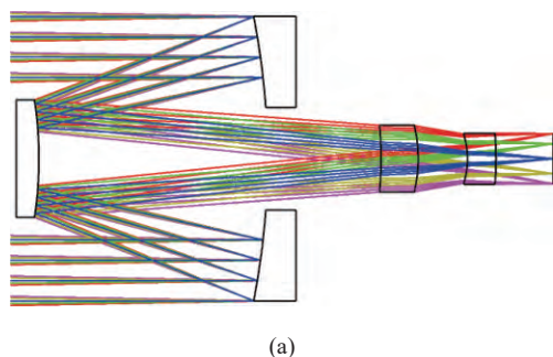
图 5 2° 视场包含两片校正镜的折反射光学系统。(a) 布局图; (b) MTF 图
