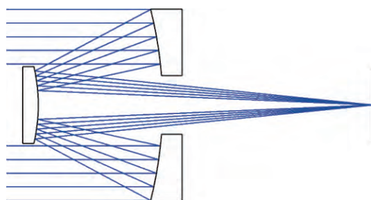
图 4 同轴两反光学系统初始系统布局图
