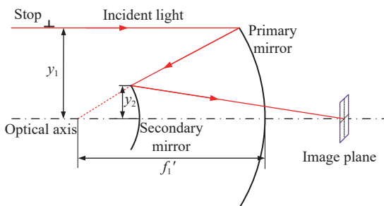
图 3 同轴两反射镜光学系统
