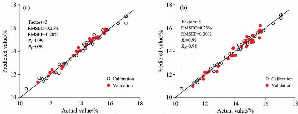
图 2 模型 I 和 II 的定标结果 Fig 2 Calibration results of model I and model II
