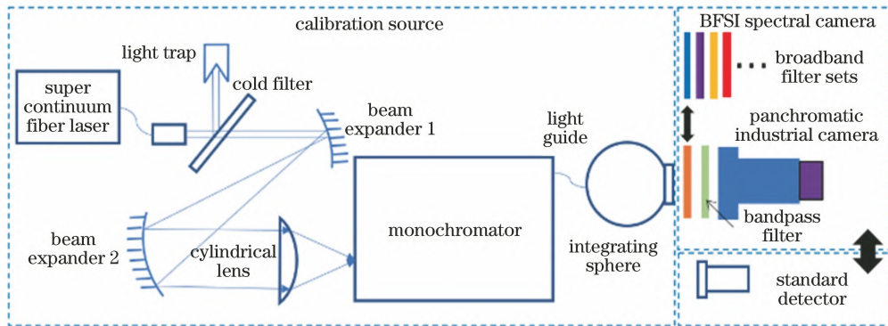
图 4 原理样机标定光源与标定过程
