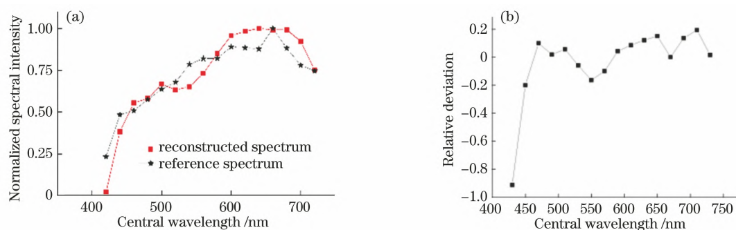
图 7 重建光谱与标准光谱的对比及二者相对偏差。(a)重建光谱与标准光谱的对比;(b)相对偏差
