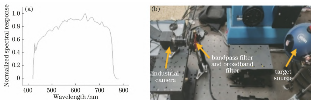
图 5 原理样机的光谱响应及原理样机的实物。(a)光谱响应;(b)原理样机装置
