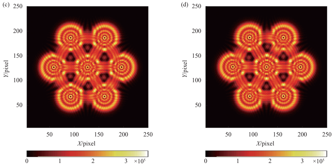
图 4 小幅值波前倾斜感知效果。(a) 倾斜波前; (b) 重建波前; (c) 焦前光强分布; (d) 焦后光强分布
