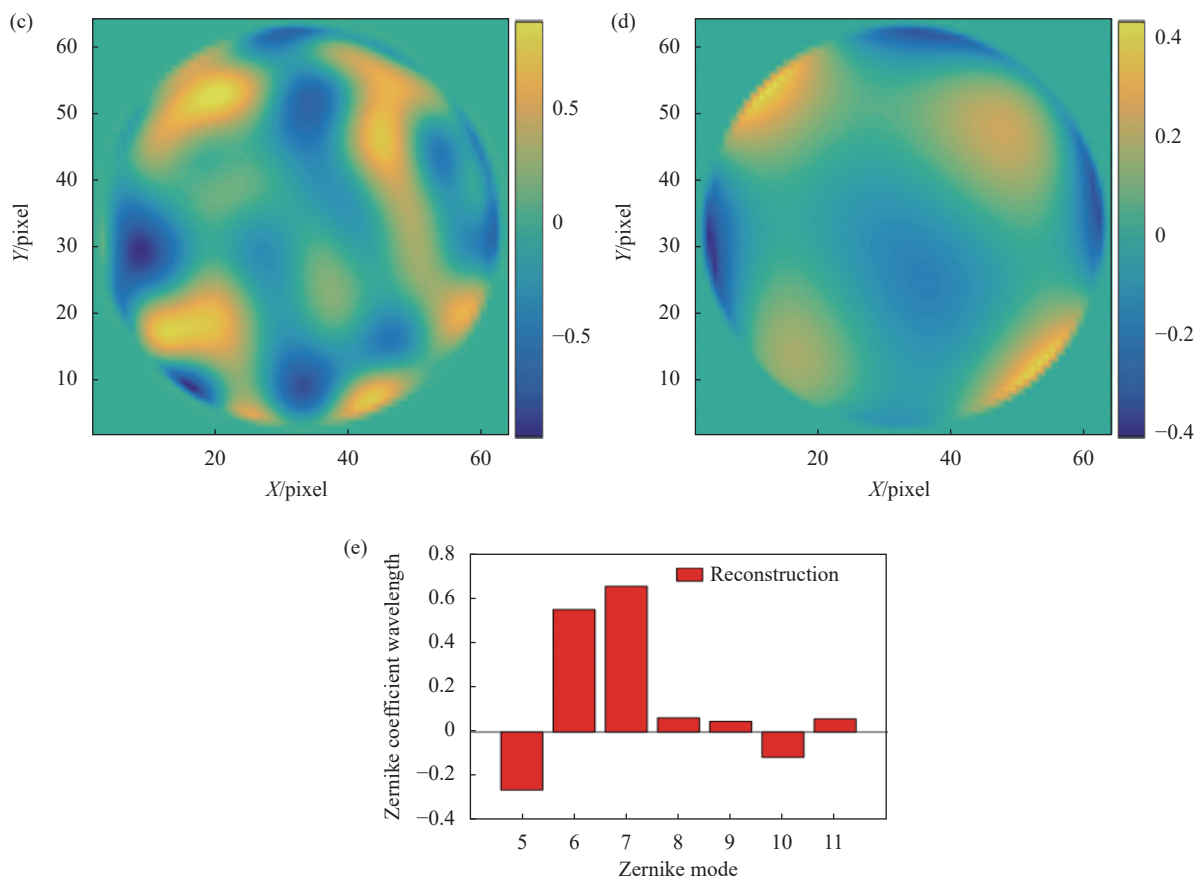
图 7 利用变形镜对边界异变感知验证结果。(a) 焦前光强分布; (b) 焦后光强分布; (c) 波前解算结果; (d) 低阶像差; (e) 低阶像差估计
