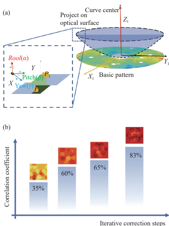
图 9 闭环校正过程。(a) 系统示意图; (b) 焦前焦后的光强差
