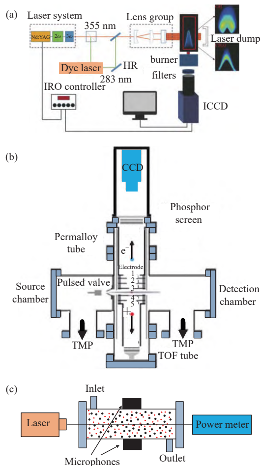
图1 转化吸收光谱技术原理图。(a)激光诱导荧光技术; (b)共振增强多光子电离技术; (c)光声光谱技术
