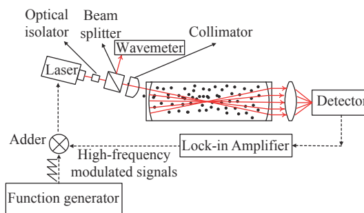
图 7 波长调制离轴积分腔光谱测量系统原理图 [35]
