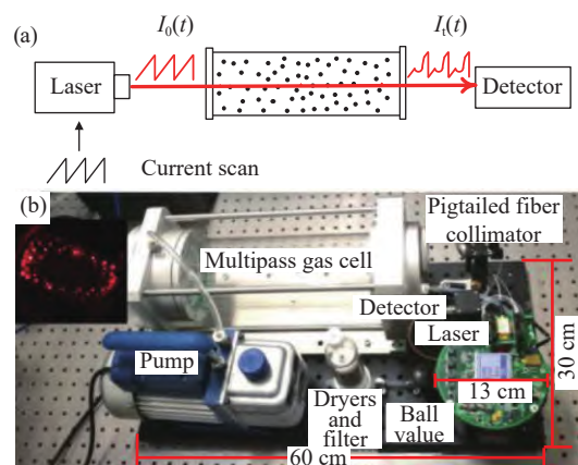
图 4 (a)直接吸收 TDLAS 技术原理图;(b)多通池 TDLAS 技术的实验装置图 [16]
