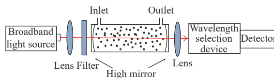
图 8 宽谱腔增强吸收光谱技术装置示意图
