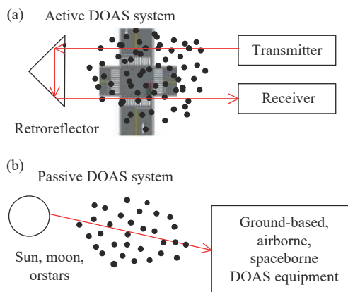
图 5 (a) 主动 (b) 被动差分吸收光谱技术示意图
