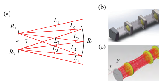
图 6 (a) White 腔原理图 [32] 。平面光学多通池的 (b) 三维结构图及 (c) 仿真模型 [34]
