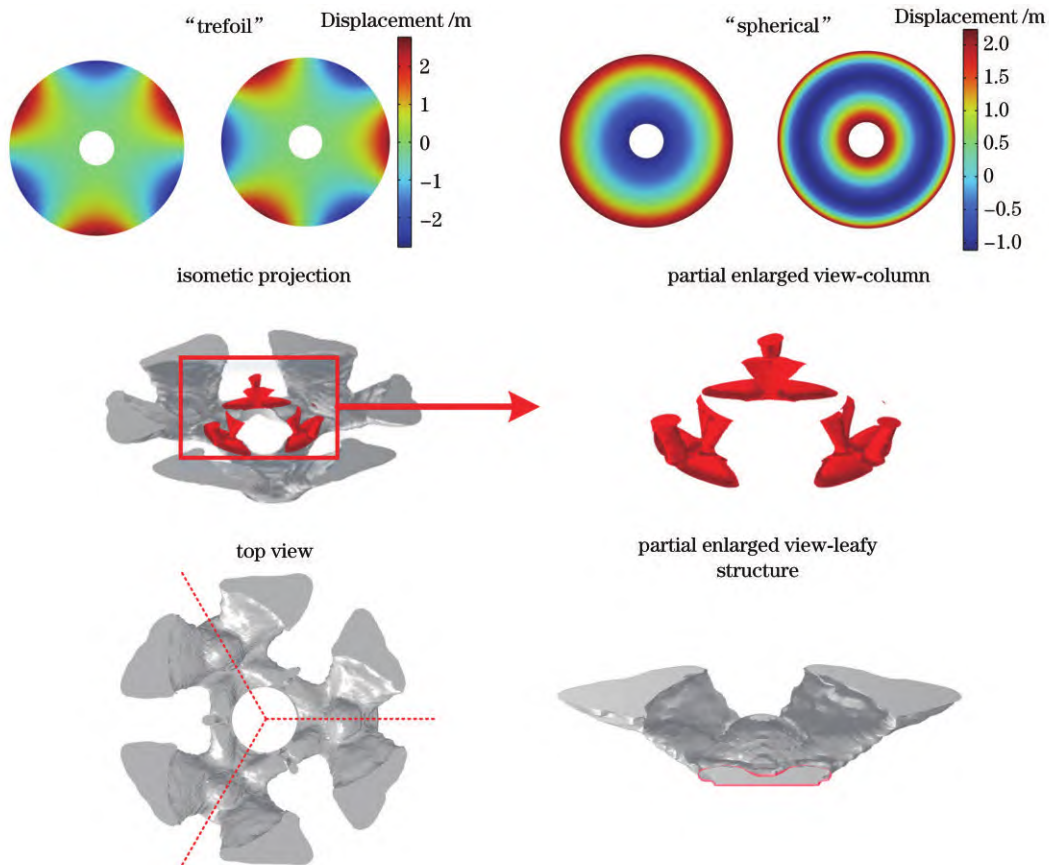
图 9 Zernike 优化结果
