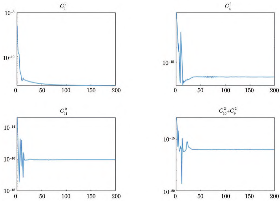
图 11 Zernike 优化稳定性 Fig. 11 Zernike optimized stability
