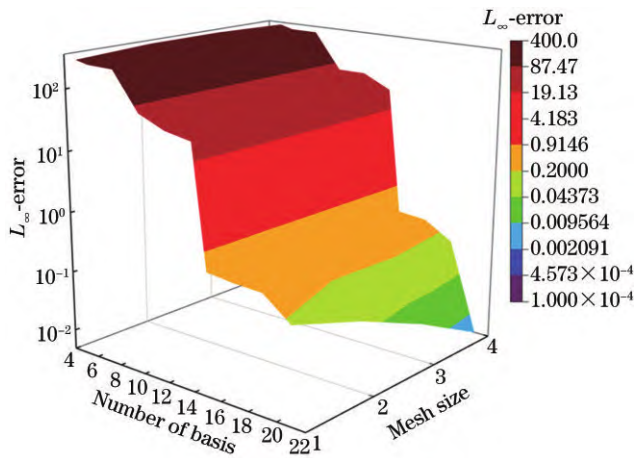
图 4 拟合误差的无穷范数
