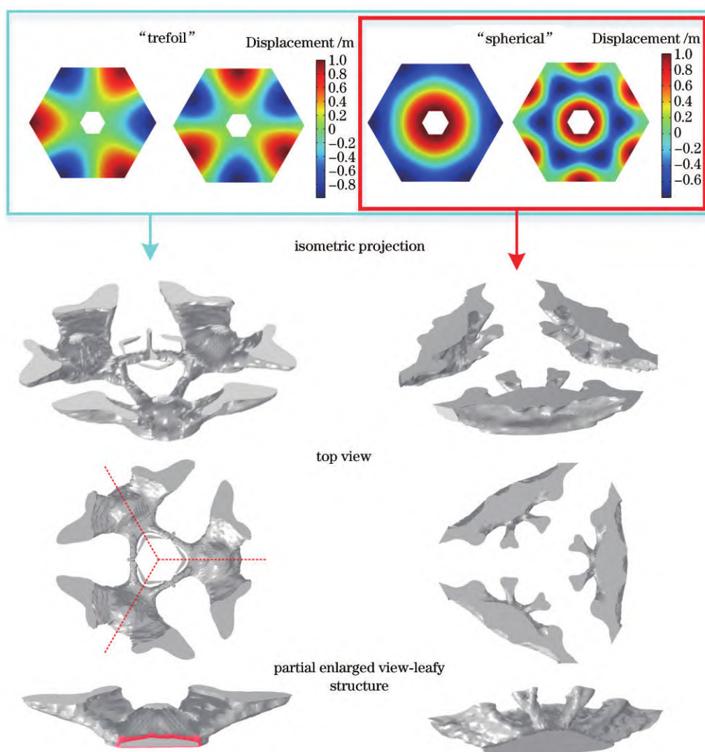
图 14 六边形镜子优化结果
