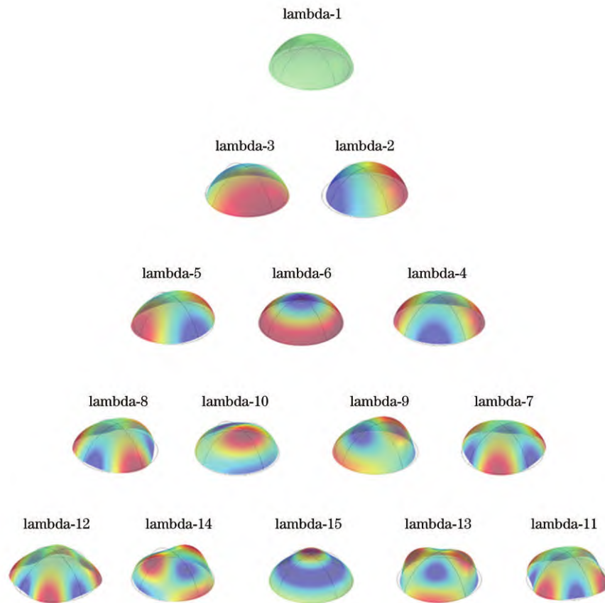
图 3 球冠特征模态
