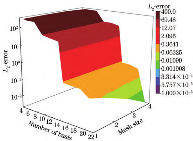
图 5 拟合误差的 2-范数
