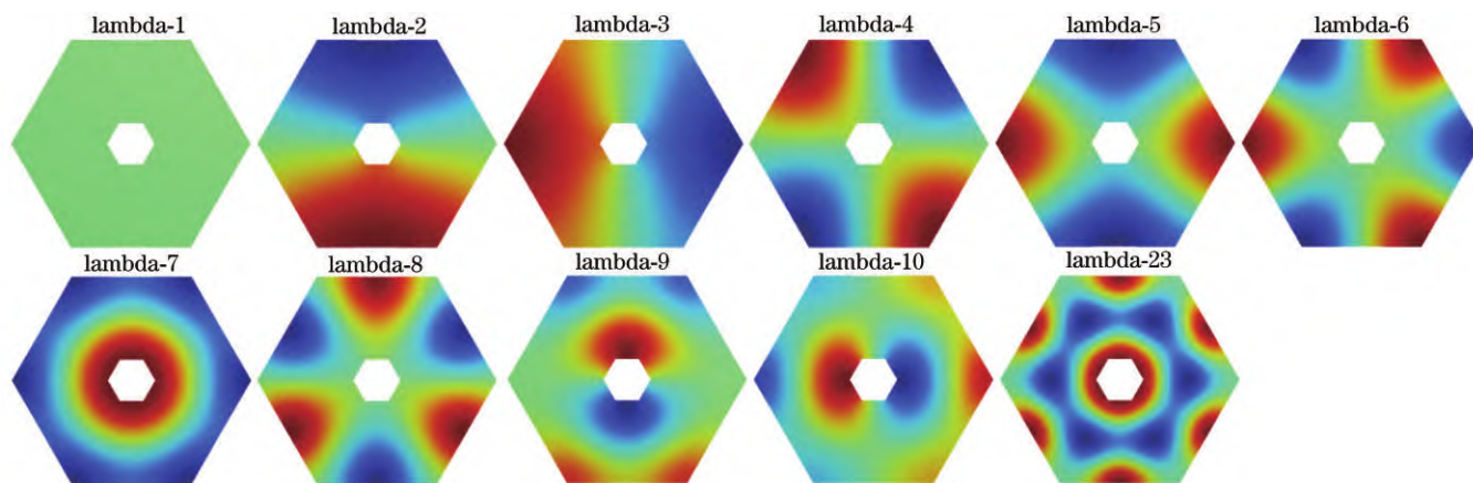
图 13 六边形抛物面特征模态
