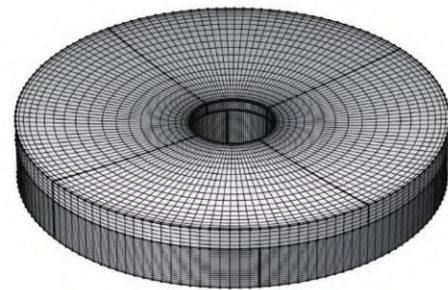
图 6 圆形镜子
