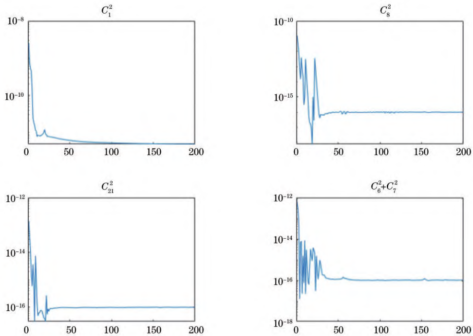
图 11 Zernike 优化稳定性 Fig. 11 Zernike optimized stability
