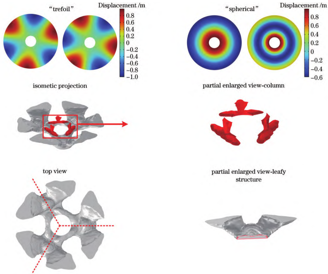
图 10 特征模态优化结果 Fig. 10 Eigenmode optimization results
